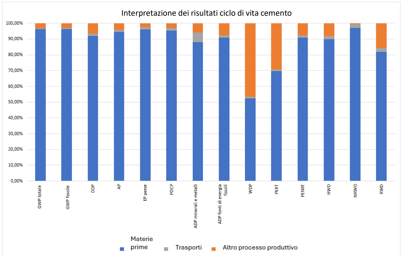
Figura 4: Analisi di dominanza della produzione di CEM II/B-LL 32,5 R
